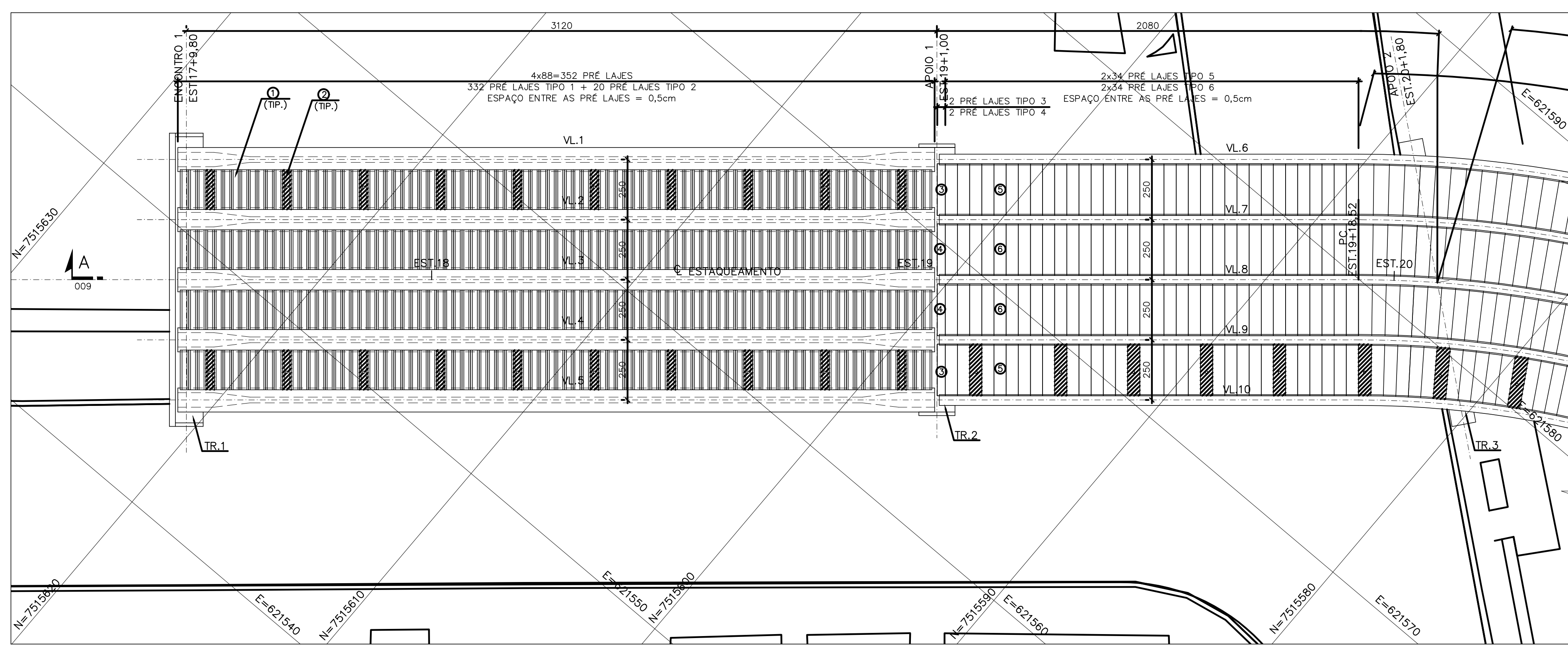
LOCAÇÃO DAS PRÉ LAJES - PLANTA - (1ª PARTE) ESC 1:125
