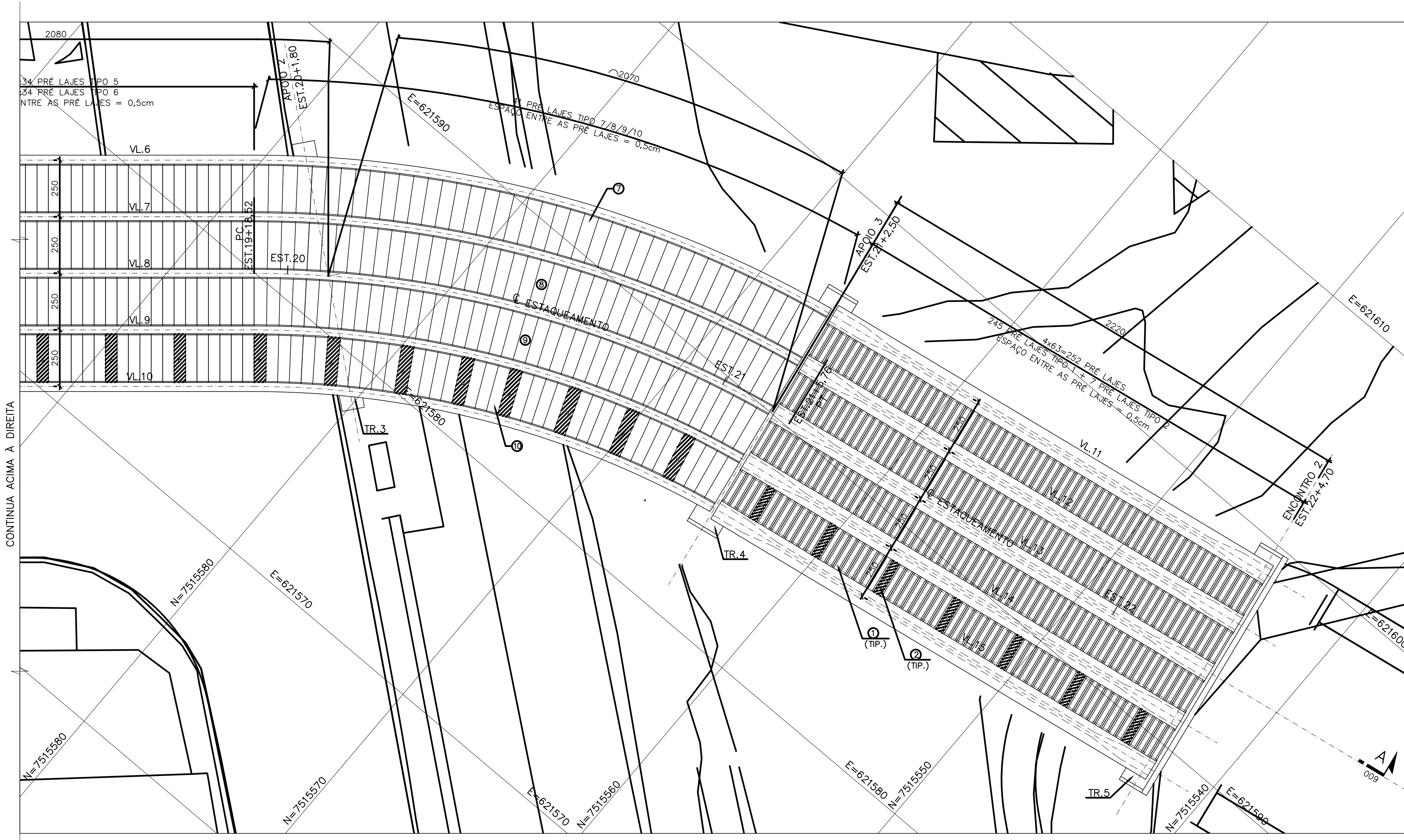
LOCAÇÃO DAS PRÉ LAJES - PLANTA - (2ª PARTE) ESC 1:125
